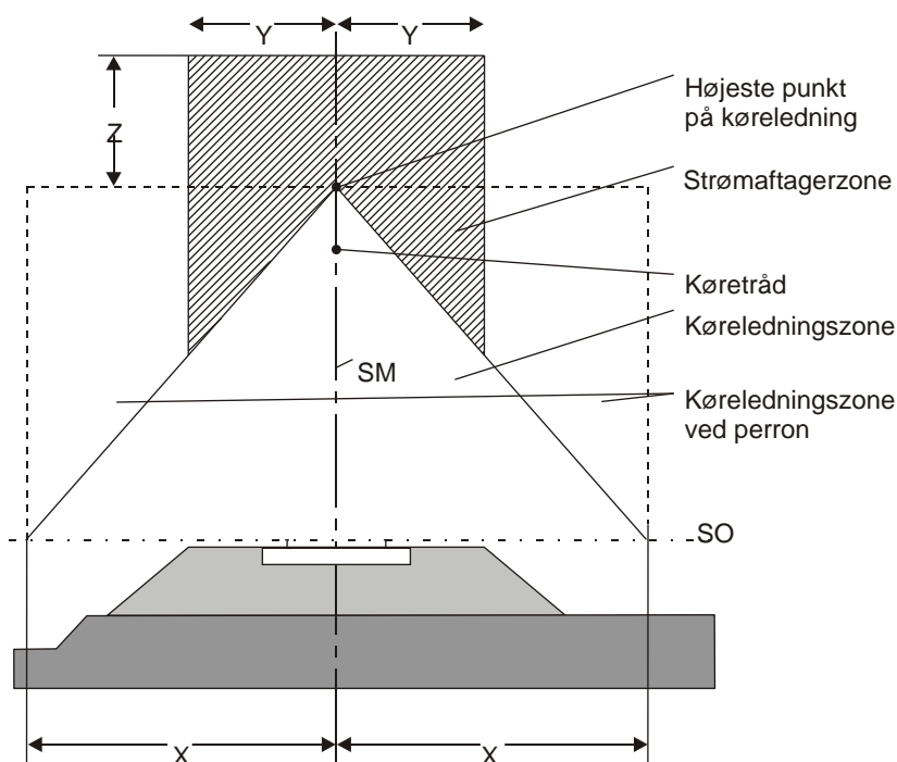
Figur 11.1-1: Køreledningszone og strømftagerzone.
