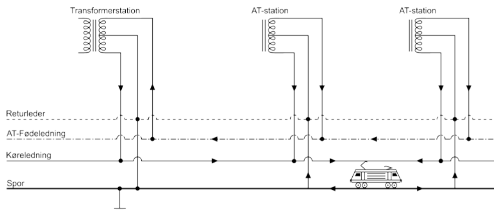
Figur Bilag 1.2: Principskema.
