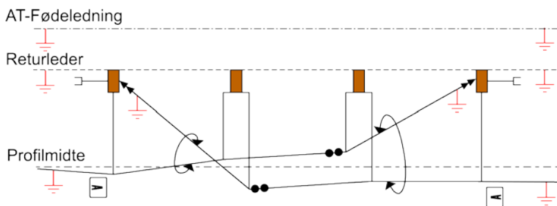
Figur bilag 10-1 Adskillelsesfelt uden ledningskobler.
