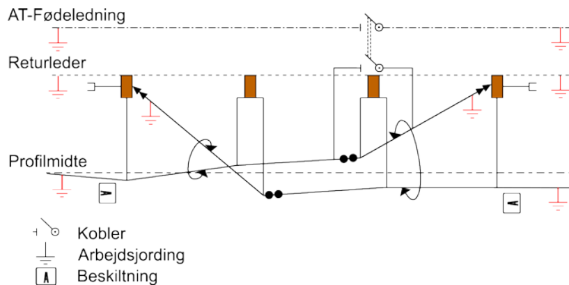
Figur bilag 10-2 Adskillelsesfelt med ledningskobler. Skilte
