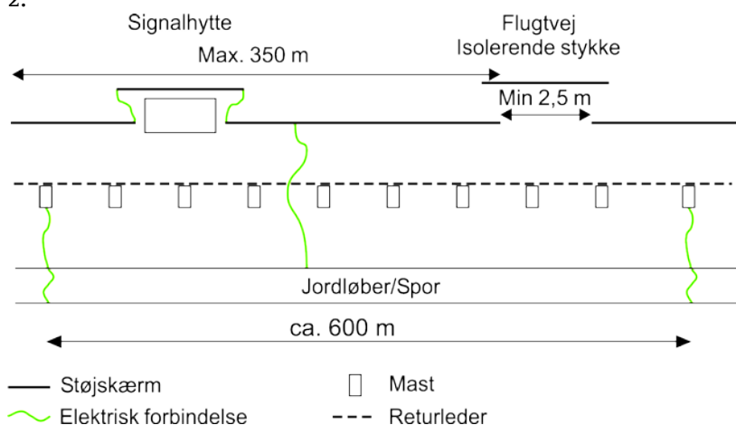
Figur 10.4.7-2 Eksempel på isolerende sektion i støjskærm.
