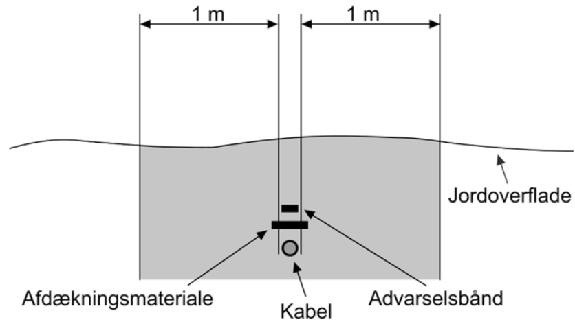
Figur 16.5-1: Kabler i jord
