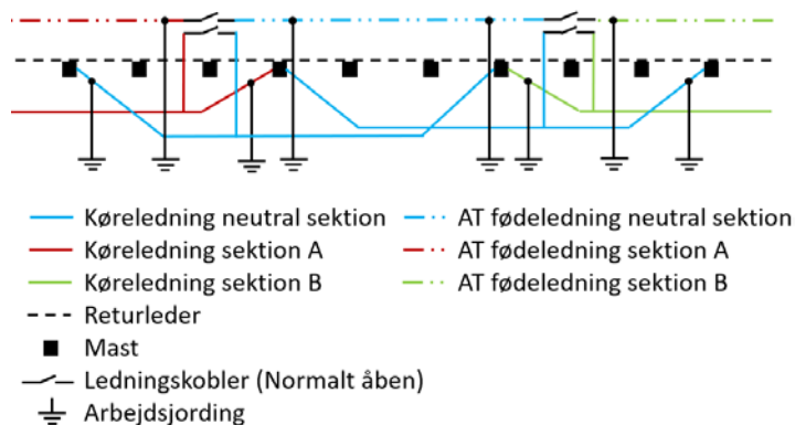
Figur 11.8.1-2 Arbejdsjording i "split" neutralsektion.
