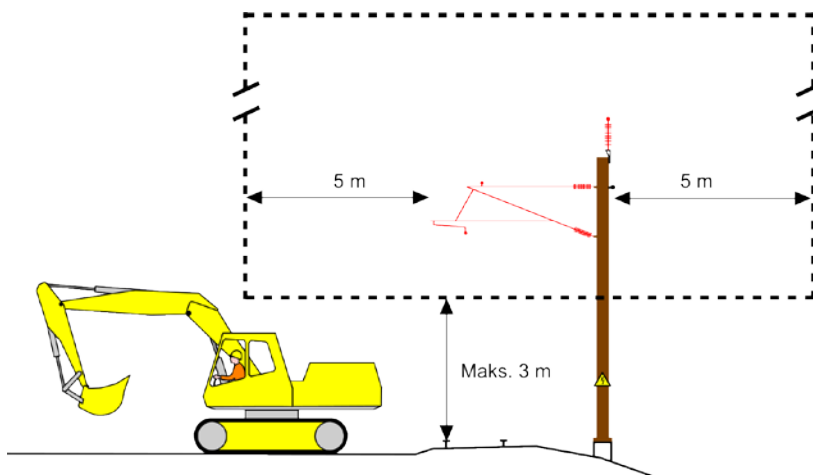
Figur 10.3.8-1 Vandret og lodret respektafstand
