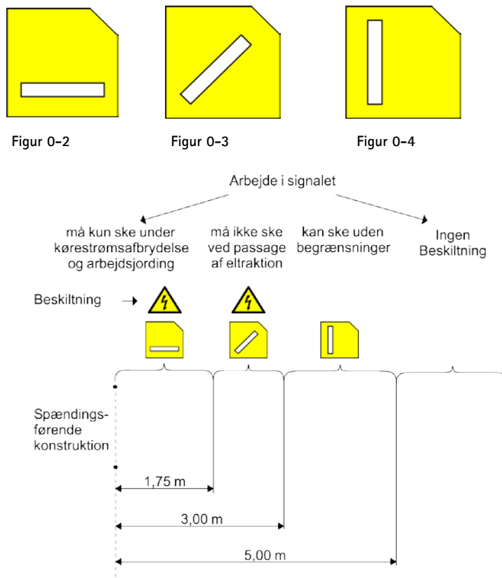
Figur 0-5 Betydning af beskiltning.
