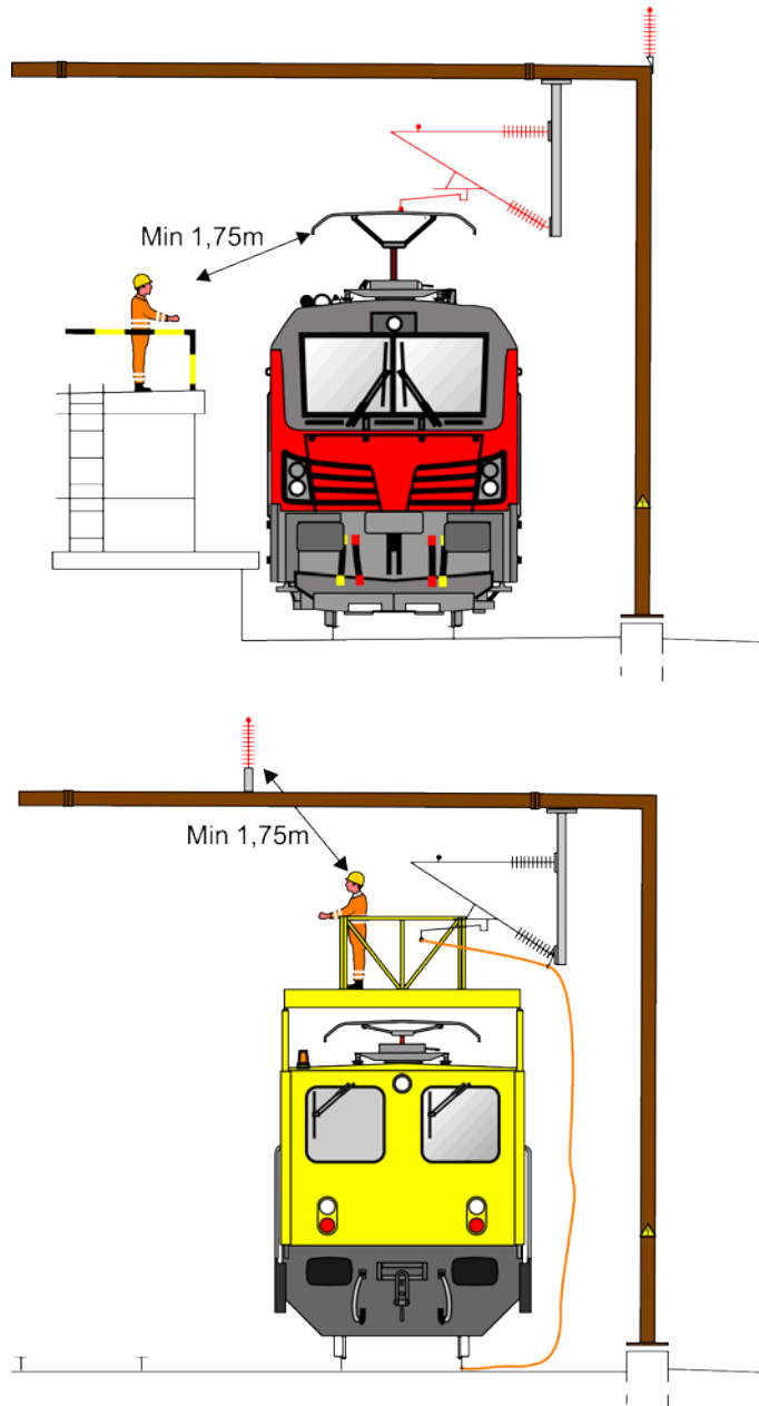
Figur 10.3.1-1 Respektafstande for personer.
