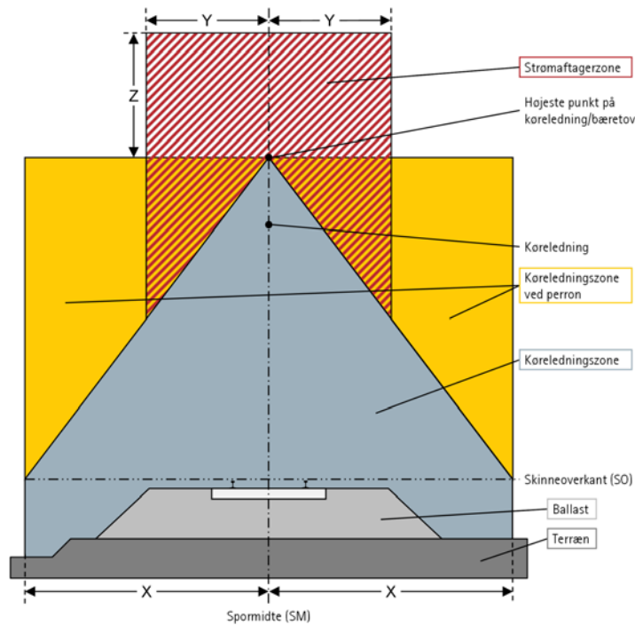
Figur 10.4.1-1 Profil af køreledningszonen og strømaftagerzonen.
