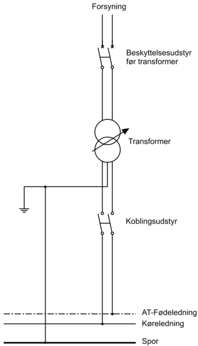
Figur 11.7-1 Princielt opbygning af en forsyningsstation med AT-Fødeledning.
