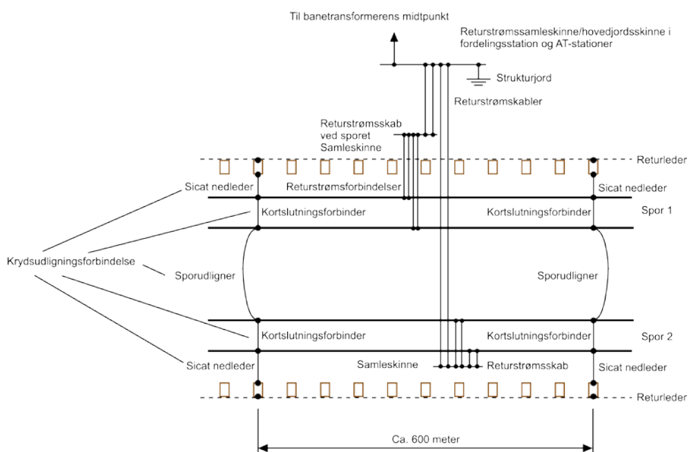
Figur Bilag 8.1-1 Principdiagram for returstrømsforbindelsernes/-kablernes tilslutningspunkter for et dobbeltspor.
