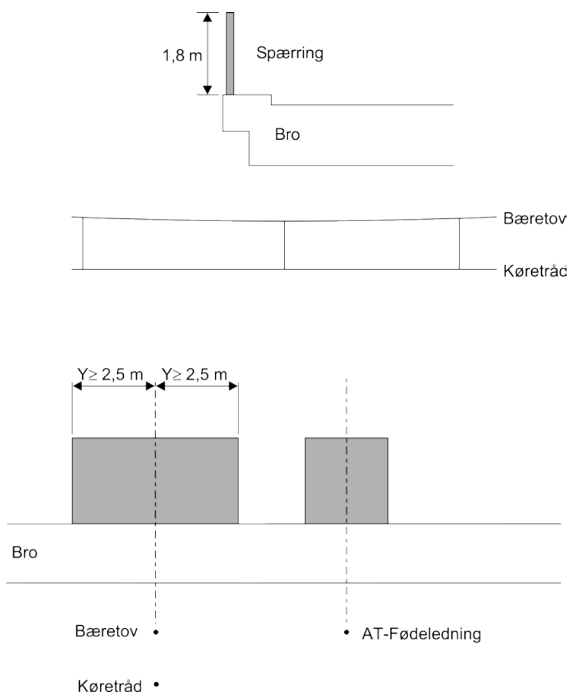
Figur Bilag 1.7:-1 Eksempel på spærring på bro.
