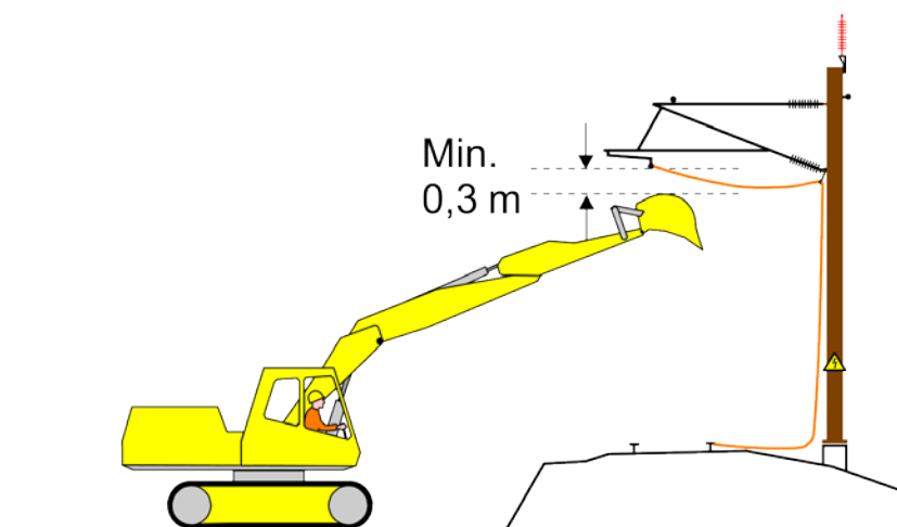
Figur 10.2.2.2-1 Mindste afstand for maskiner og værktøj.
