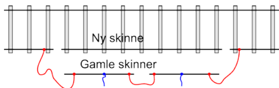
Figur 12.2.8.1-1 Rødmarkerede kabler er midlertidige kabelforbindelser (overstropninger), blåmarkerede kabler er returstrøms- eller potentialudligningsforbindelser.
