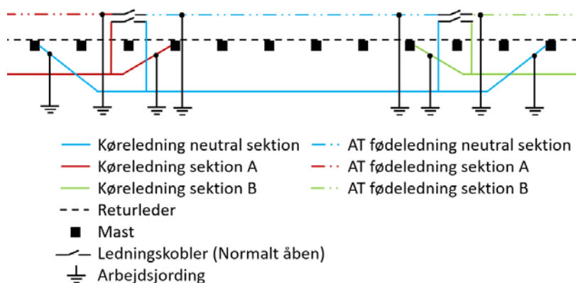
Figur 11.8.1-1 Arbejdsjording i lang neutralsektion.
